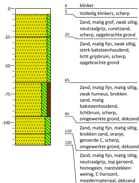
Boring: 016
